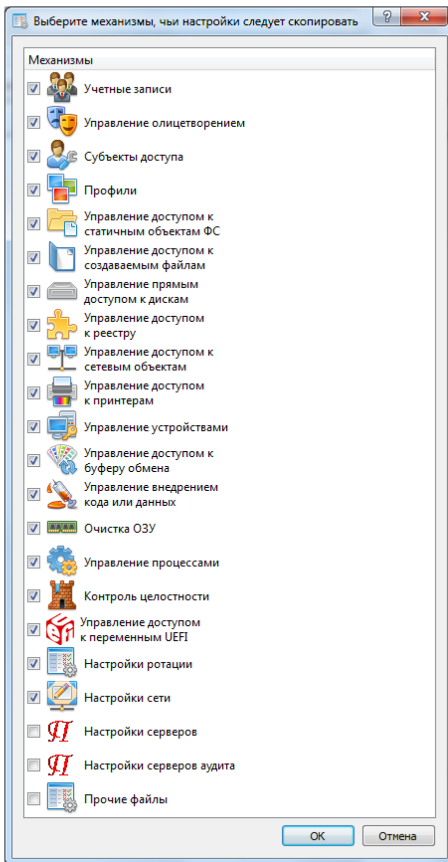
Рис.2.4. Выбор механизмов защиты, настройки которых должны быть скопированы
